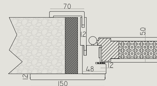
TELAIO - FRAME - CADRE - Коробка PREMIER EI 30 CAPITELLO - CAPITAL - CHAPITEAU - КАПИТЕЛЬ II7
