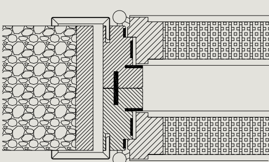
Porta comunicante Interconnecting door Porte de communication Сдвоенные двери
