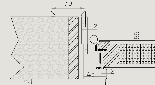
TELAIO - FRAME - CADRE - Коробка PREMIER EI 60 CAPITELLO - CAPITAL - CHAPITEAU - КАПИТЕЛЬ II7
